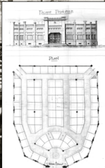
Projet de plan de la façade des halles
