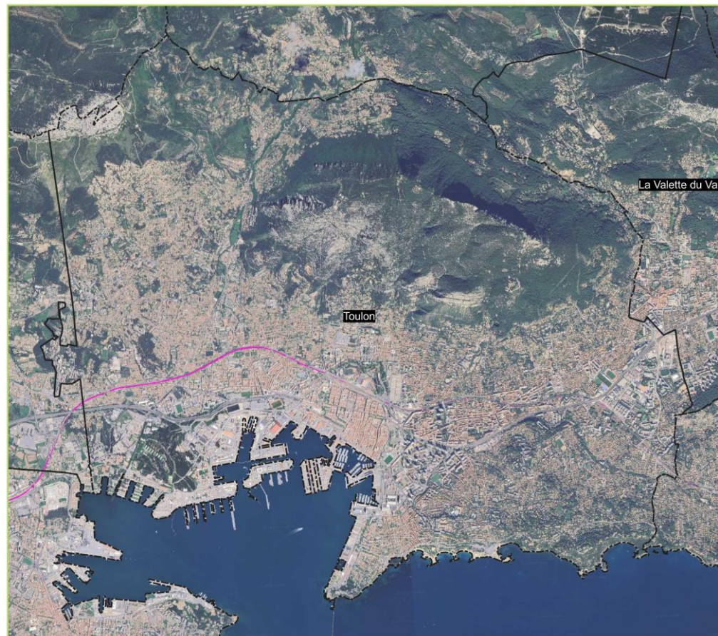
Carte de Bruit Stratégique "Type C" Isophone Ln Bruit ferroviaire
