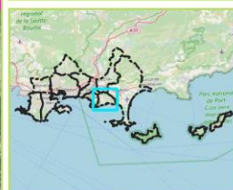
Carte de Bruit Stratégique "Type C" Isophone Ln Bruit routier
