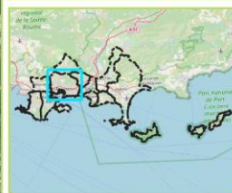
Carte de Bruit Stratégique "Type C" Isophone Lden Bruit ferroviaire
