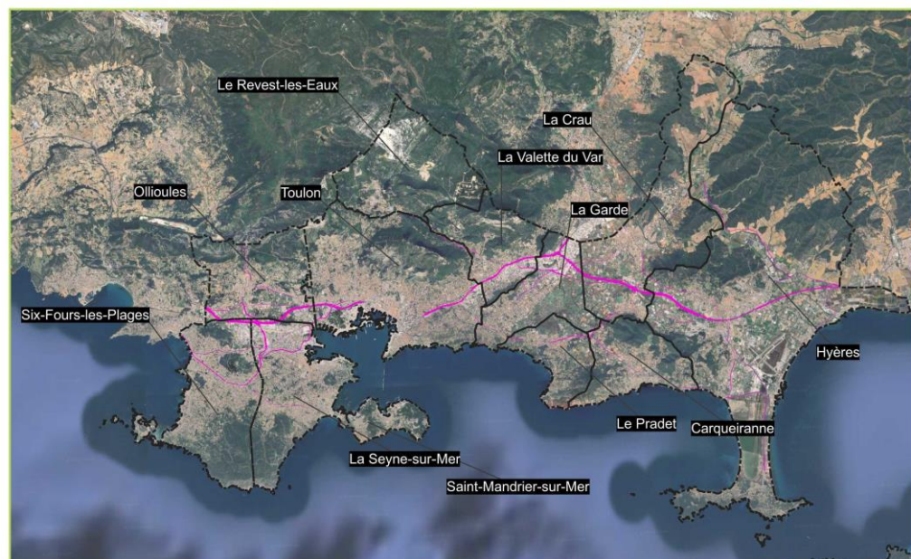
Carte de Bruit Stratégique "Type C" Isophone Ln Bruit routier
