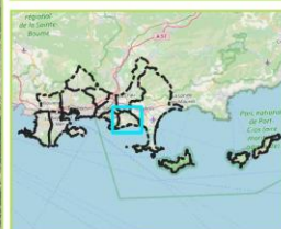
Carte de Bruit Stratégique "Type C" Isophone Ln Bruit ferroviaire
