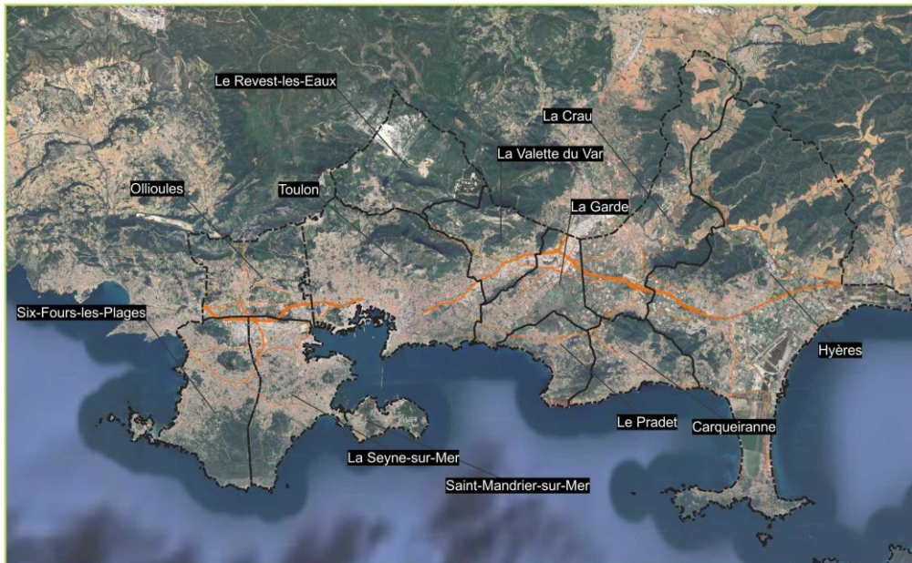
Carte de Bruit Stratégique "Type C" Isophone Lden Bruit routier
