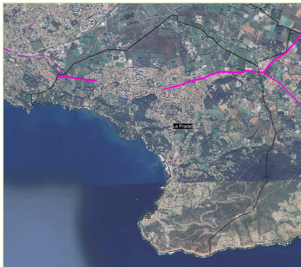
Carte de Bruit Stratégique "Type C" Isophone Ln Bruit routier
