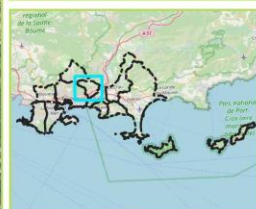
Carte de Bruit Stratégique "Type C" Isophone Lden Bruit routier
