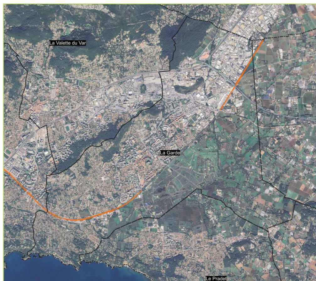
Carte de Bruit Stratégique "Type C" Isophone Lden Bruit ferroviaire
