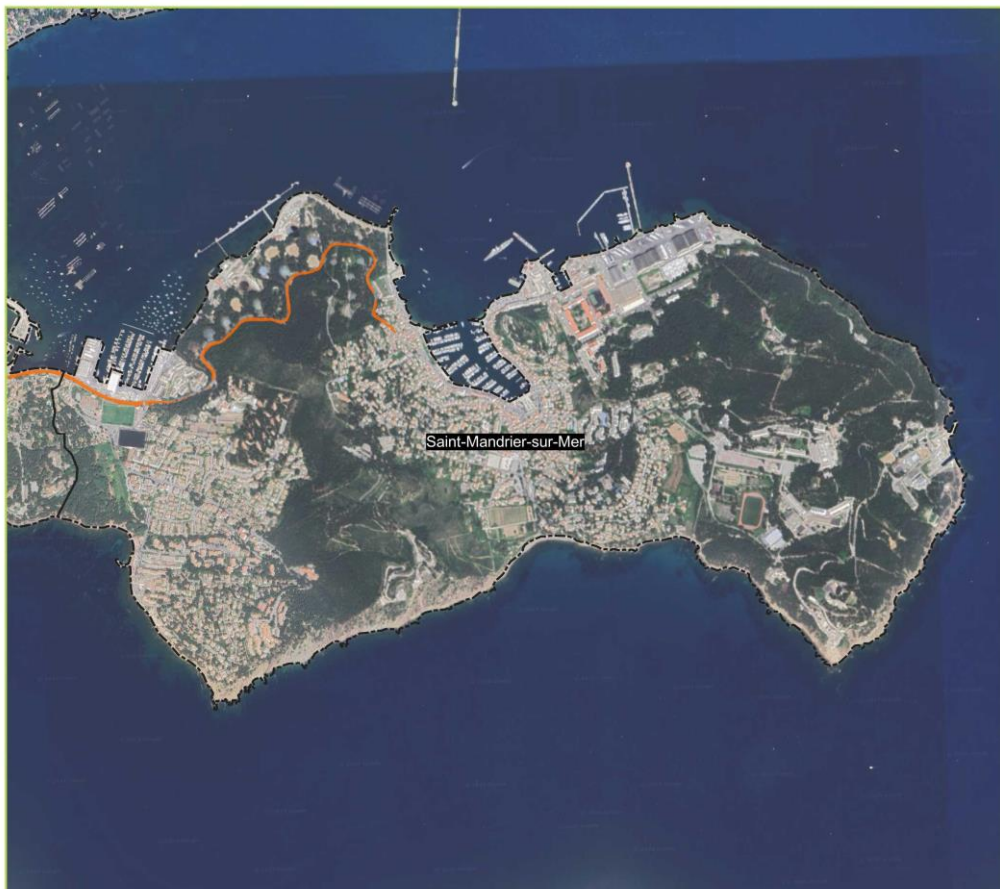
Carte de Bruit Stratégique "Type C" Isophone Lden Bruit routier
